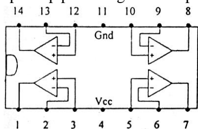
Gambar 12. Op-Amp dalam rangkaian IC (Wikipedia.com)
