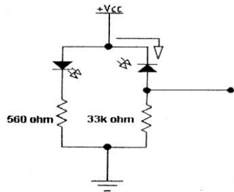
Gambar 16. Sensor tidak terkena Cahaya (Wikipedia.com)
