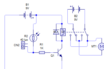
Gambar 2. Pembuatan Driver Relay (Dokumentasi Pribadi)
